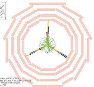
Τροχιές και πίδακες στοιχειωδών σωματιών (Γεγονός του πειράματος CMS στο CERN)
